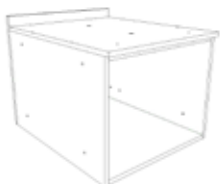
MB104 - Open Void 637(L) x 800/950(W) x 519(H)
